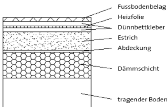
Wärmedämmung und Verlegung als Flächen-, Direktheizung im Dünnbettkleber.
